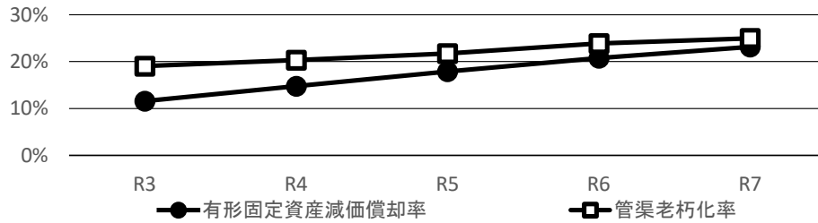
有形固定資産減価償却率・管路老朽化率の推移
