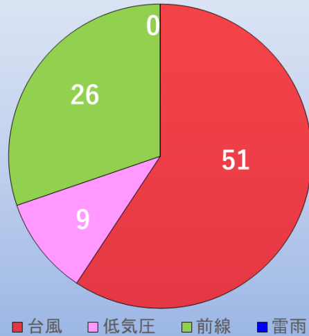
内水排除要因【改築前】
