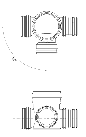
図 2-8 硬質塩化ビニル製リブ付小型マンホール用インバート
