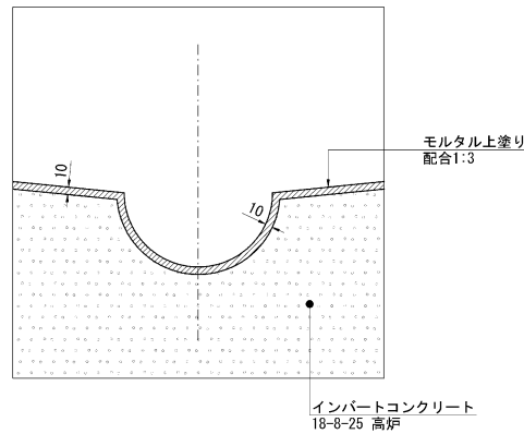
図 2-4 インパート施工図
