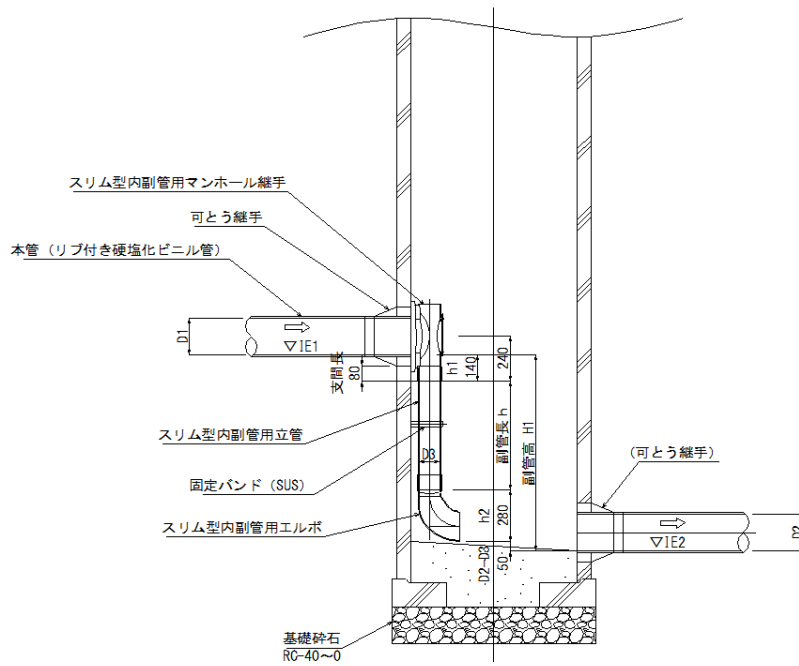
図 2-5 内副管標準図
