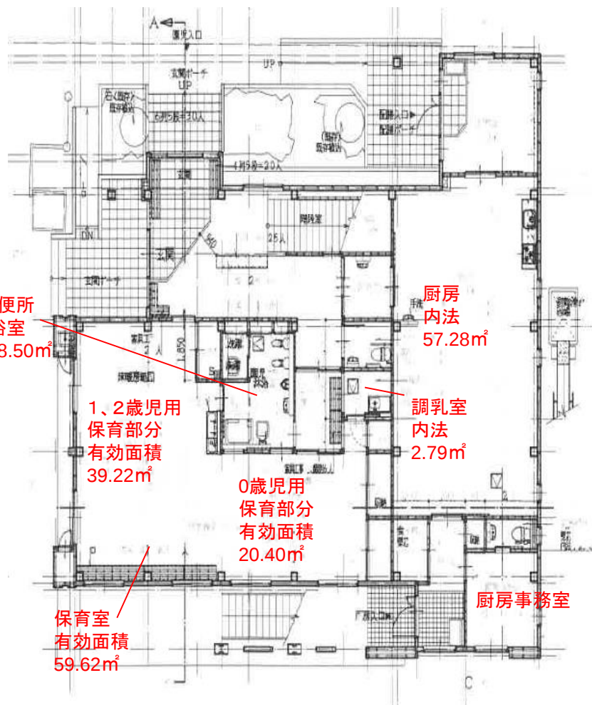
1階
