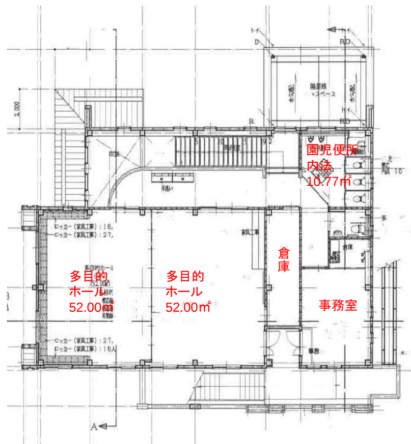
2階
