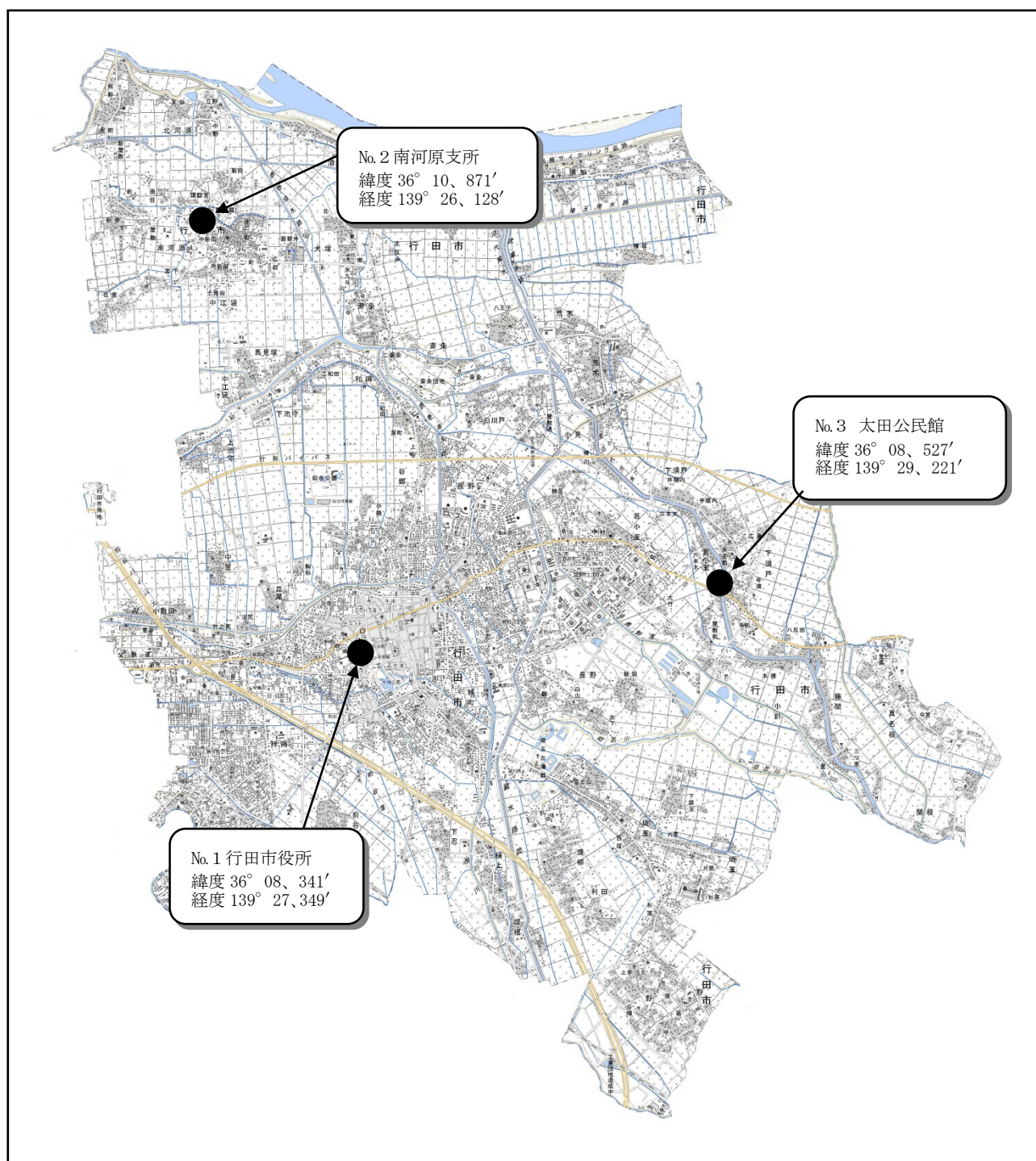
図1 令和7年度行田市における大気中のダイオキシン類調査箇所
