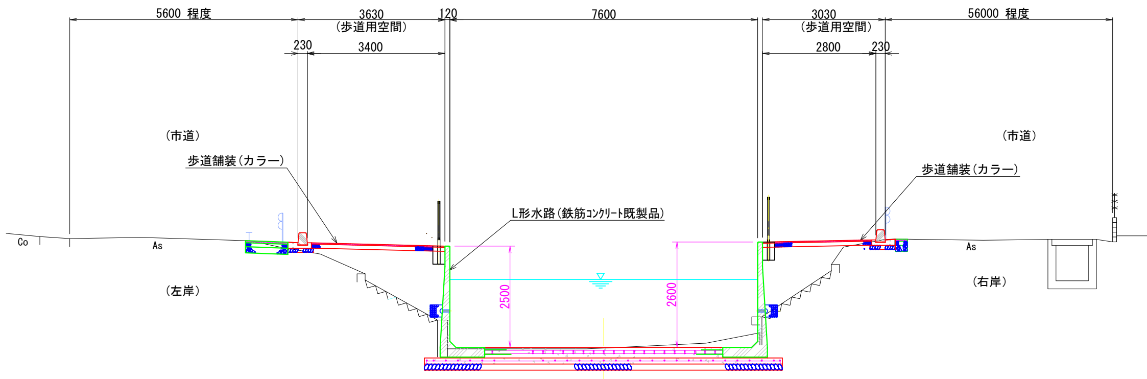
標準断面図 S=1:100
